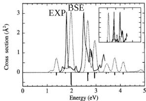
Sodium tetramer
